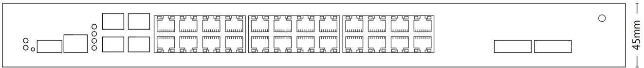
440mm 前视图
